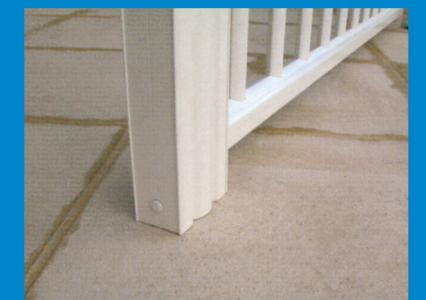
Fijación en tubo empotrable
