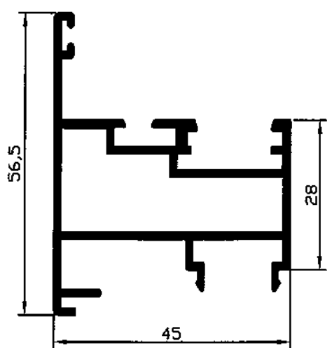
4504 Perfil inversor
