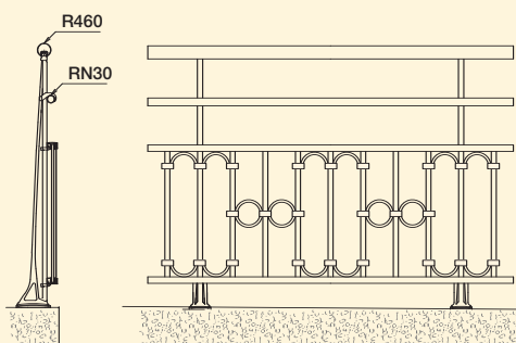
VERSION VIDE SOUS MAIN COURANTE AVEC 1 LISSE INTERMÉDIAIRE
