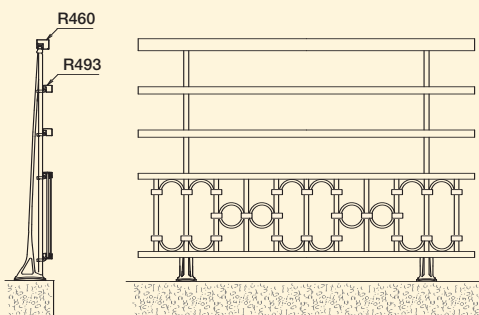
VERSION VIDE SOUS MAIN COURANTE AVEC 2 LISSES INTERMÉDIAIRES
