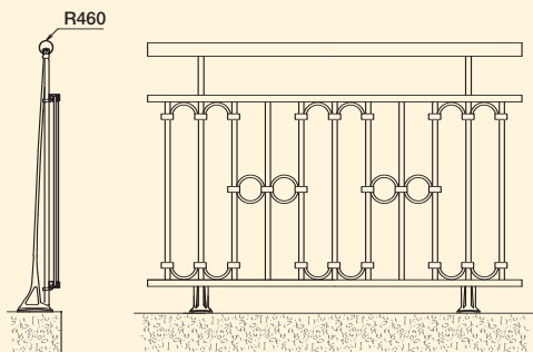
VERSION VIDE SOUS MAIN COURANTE
