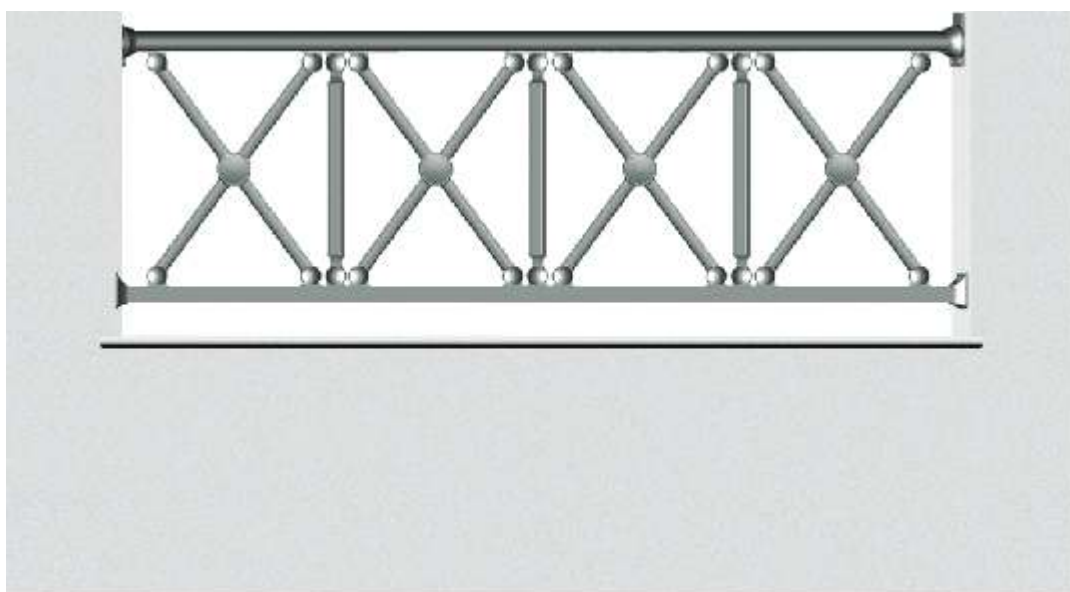
MAK-12+MAK-5-350 (Altura 50 cm) Barrotes en cruz ajustables pequeños Piezas/metro: (3 MAK-12)(2 MAK-5-350)
