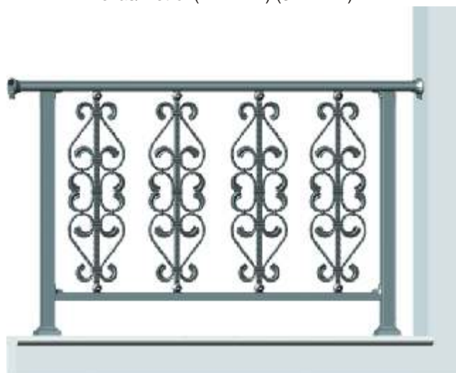
MAK-1 (Altura 80 cm) Piezas/metro: 3.3
